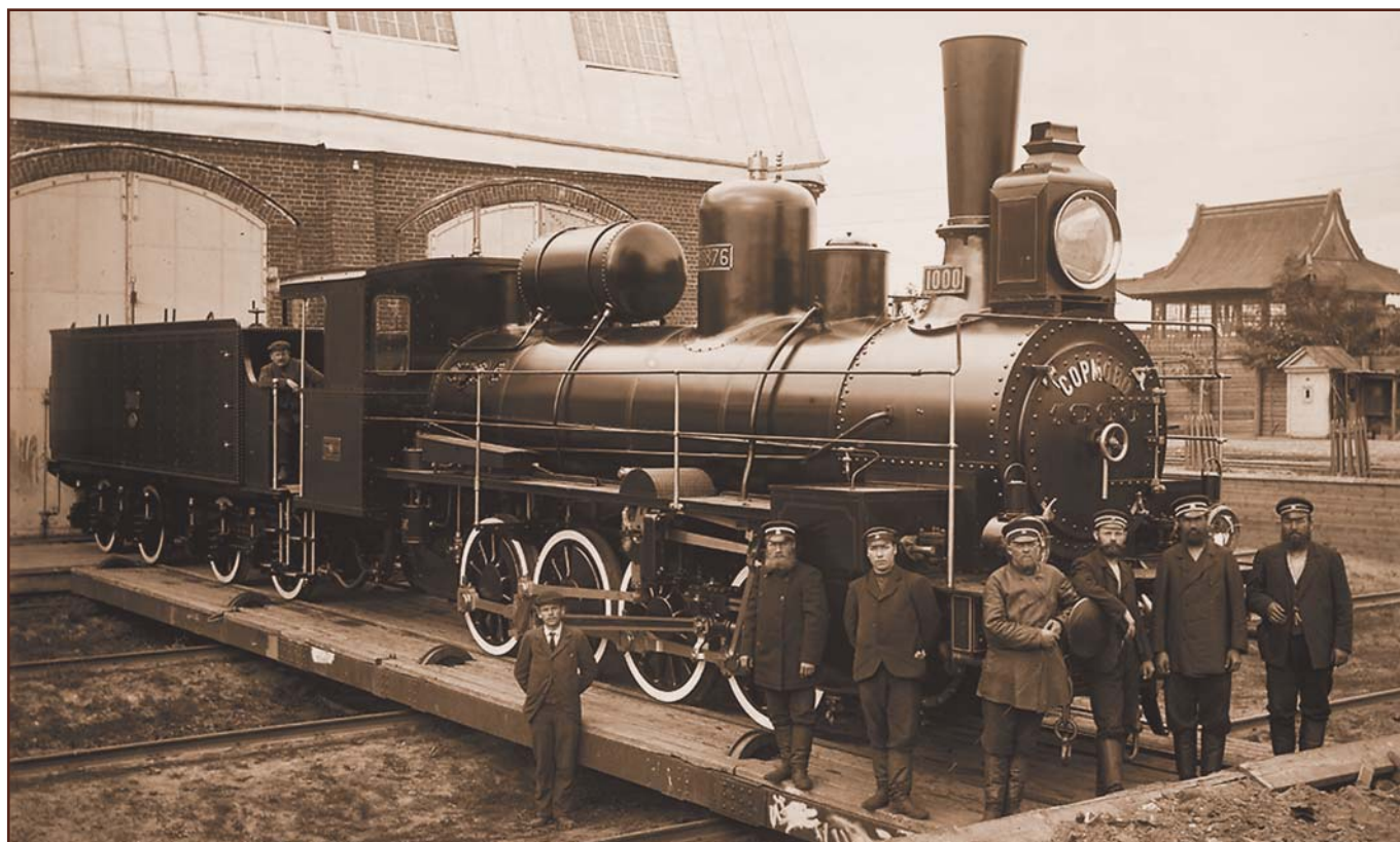
Юбилейный 100-й паровоз. Нижний Новгород, 1905 г.
